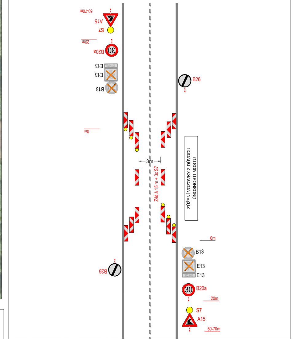
DETAIL MOSTU 352-010 SÁZAVA
